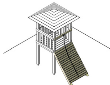
Bergsteigerrampe aus Halbrund- hölzern und mit Halteseil Fr. 850.-
