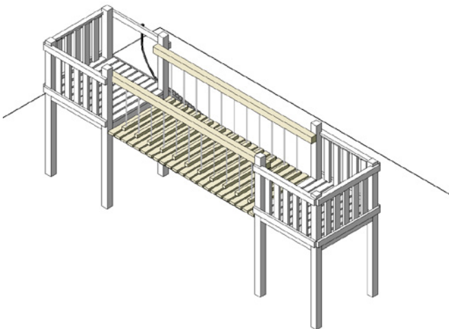
Wackelsteg 300 cm lang, mit Durchtrittschutz Fr. 2'200.- ohne Durchtrittschutz mit Eintrittsportal Fr. 1'700.- (nur bodennahe Montage)
