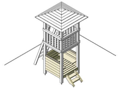
Bänkliabteil Podest mit zwei Sitzbänken, drei Täferelementen und einer kl. Treppe Fr. 1'300.- ohne Podest und ohne Treppe mit 3 Geländerelementen Fr. 840.-
